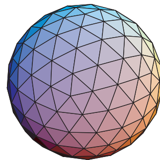
Figura 6.6. Un poliedro
