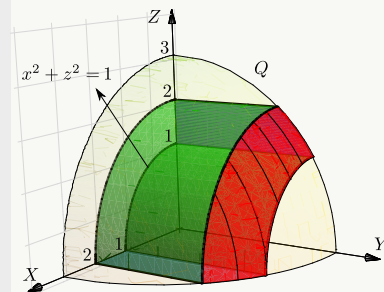
Figura 6.4. Sólido Q
